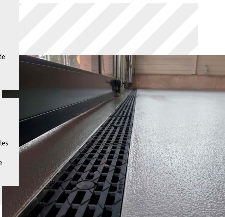
← Caniveau avec supports de montage et de pose.
