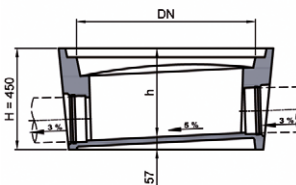
Detail Höhe 400 mm / Hauteur détail 400 mm Detail Höhe 450 mm / Hauteur détail 450 mm
