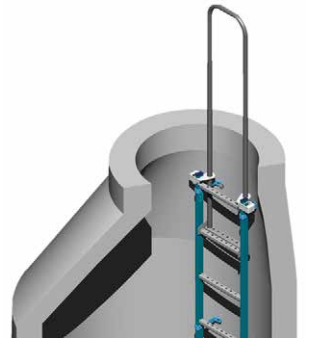
hinten laufend Coulissant par derrière
