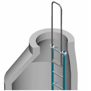
vorne laufend Coulissant par devant
