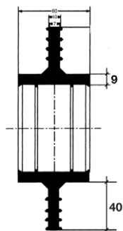
AD Rohr von 32 - 315 mm / Diam. ext. tube 32 - 315 mm AD Rohr von 355 - 1400 mm / Daim. ext. tube 355 - 1400 mm
