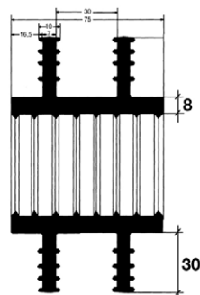
AD Rohr von 32 - 315 mm / Diam. ext. tube 32 - 315 mm AD Rohr von 355 - 1400 mm / Daim. ext. tube 355 - 1400 mm
